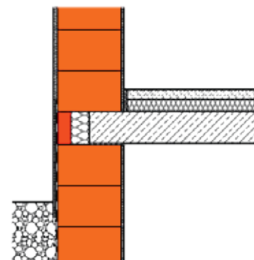
Kellerdecke Ziegelkeller
