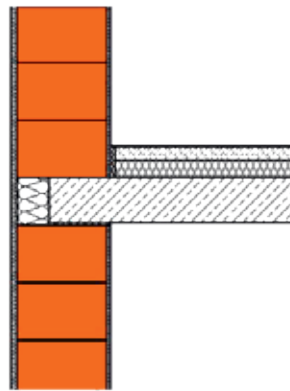
Deckenauflage MFH
