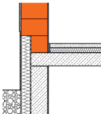
Kellerdecke Variante 2
