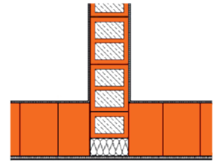
Einbindung Schallschutzwand MFH
